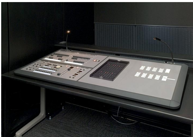
報道スタジオ 記憶調光操作卓 (パステルII)
