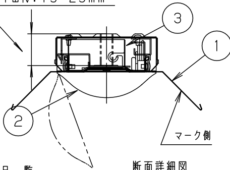
断面詳細図
