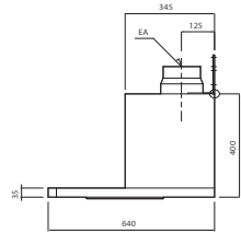
60DWD3S4.DXF
