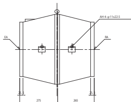
45GSV304.DXF
