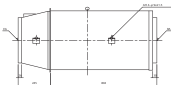
45DTH004.DXF
