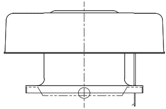
55UTL204.DXF
