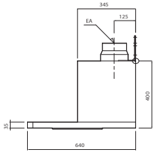
60DWA3S4.DXF
