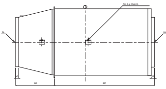
60DWA3S4.DXF
