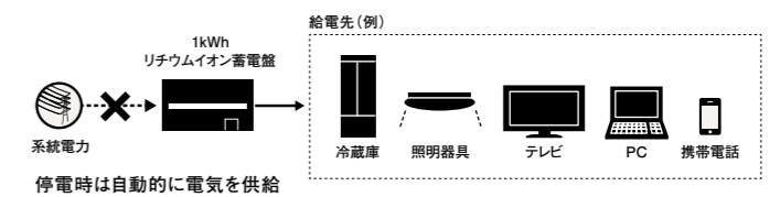
停電時の電気の流れ
