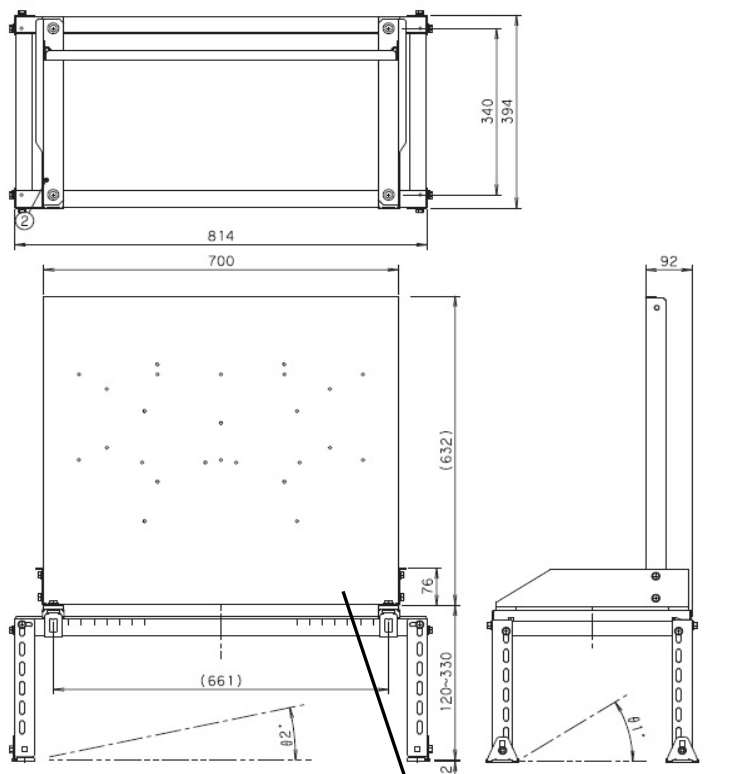
□外形寸法図
