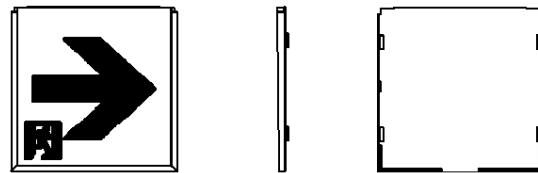
FK20017 (通路誘導灯用表示板)
