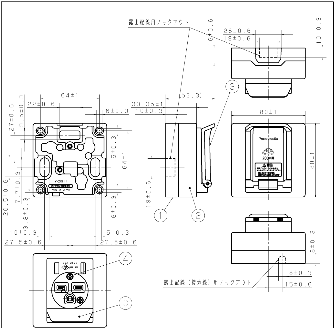
コンセントカバーを開いた状態
