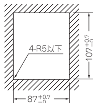
パネルカット寸法図
