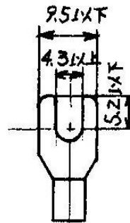
Y形圧着端子
