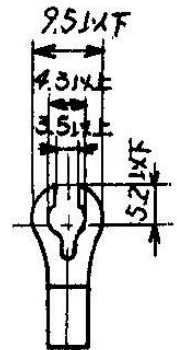
クワ形圧着端子
