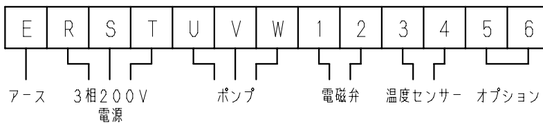
端子図
