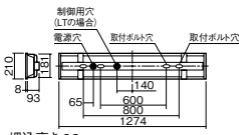
埋込高さ 93
