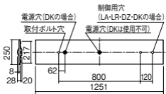
埋込高さ 20
