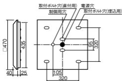
埋込高さ 25 (半埋込の場合)
