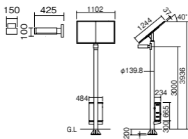
■ポール底面取付寸法図
