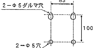
取付寸法図
