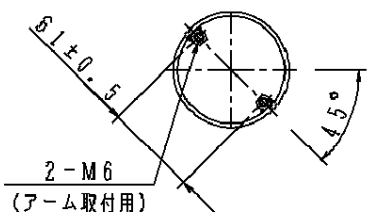
先端部詳細図 (Bから見る)
