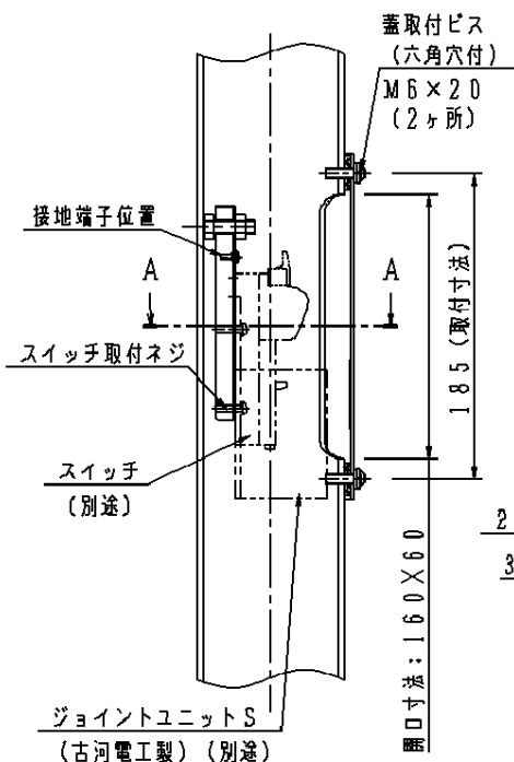
断面 A-A
