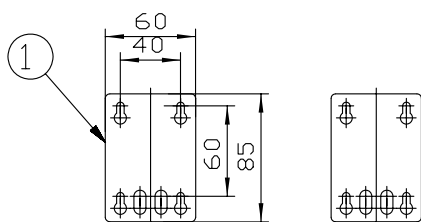
連結金具2枚
