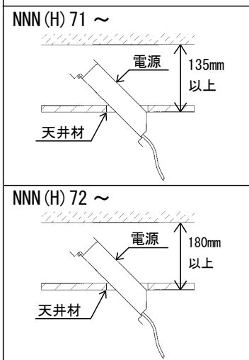
図1 埋込深さ
