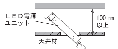
図 1 埋込深さ
