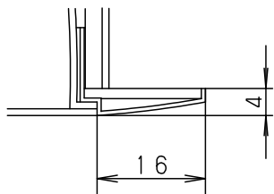
枠部詳細
