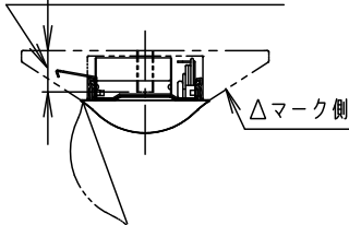
本体取付例 (NNLK41515の場合)
