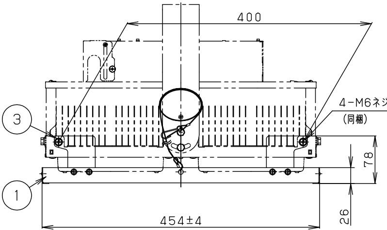
落下防止ワイヤー (SUS304, 長さ390)
