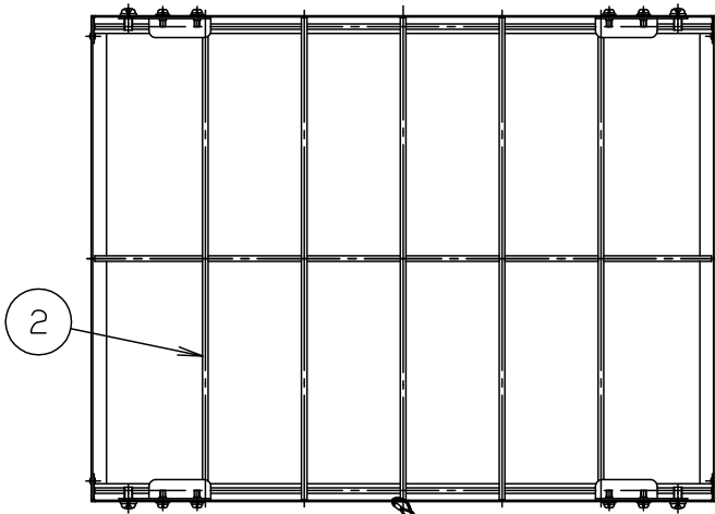
落下防止ワイヤー (SUS304, 長さ390)
