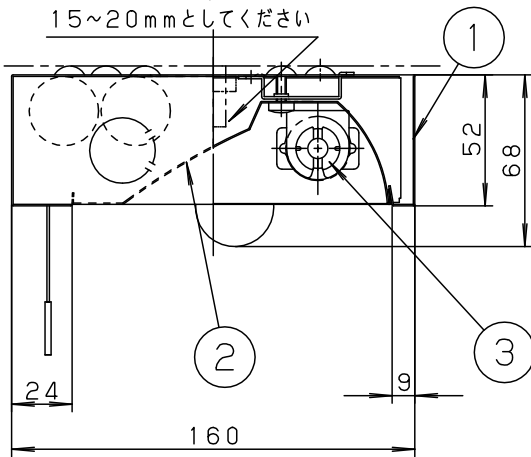
半断面詳細図
