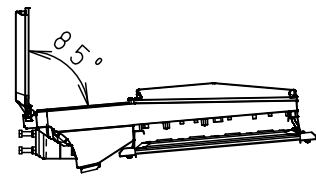
蓋開放状態
