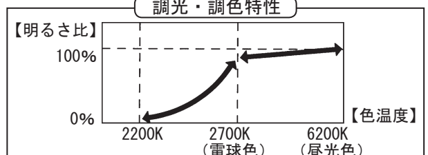
調光・調色特性
