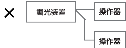
間違った配線方法
