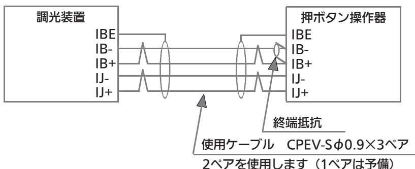
正しい配線方法
