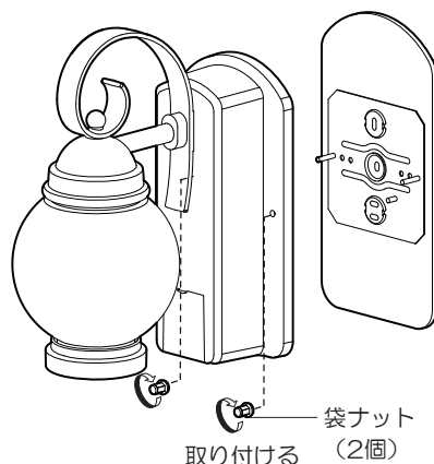
袋ナット 取り付ける (2個)
