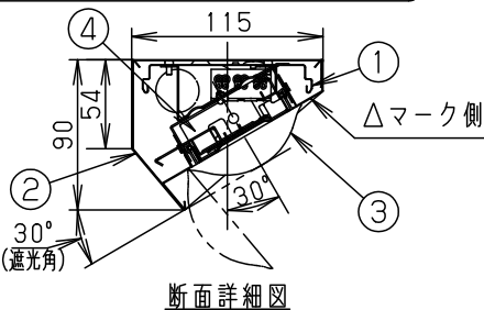
断面詳細図
