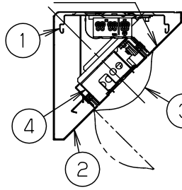
断面詳細図
