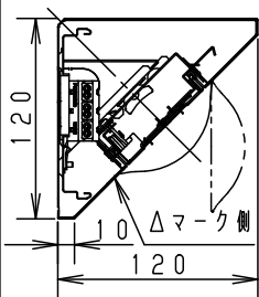
断面詳細図
