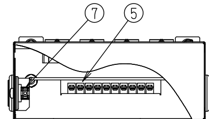
内部構成（上面側） （端子合カバー、内部配線は記載省略）
