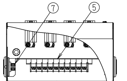
内部構成（上面側）
