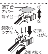
端子台カバー
