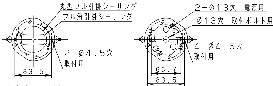
(A) 丸型フル引掛シーリングの場合 (B) ボルト又はボックスを使用する場合 フル角引掛シーリング
