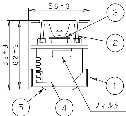
側面拡大図
