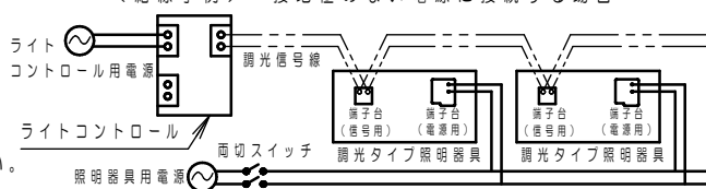
＜結線事例＞ 接地極のない電源に接続する場合
