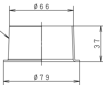
断面図 A-A
