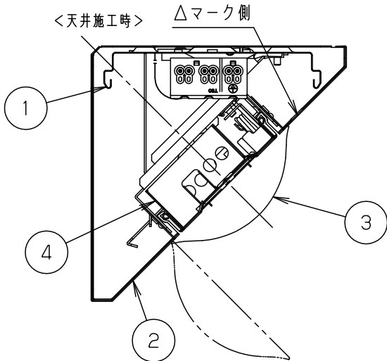
断面詳細図
