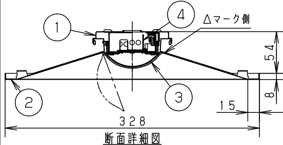
断面詳細図
