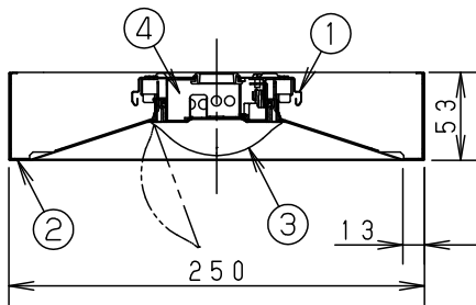
断面詳細図
