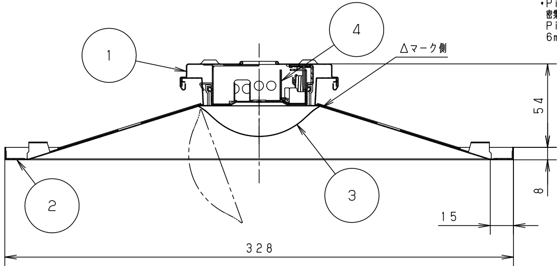
断面詳細図
