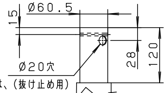
灯具前方
