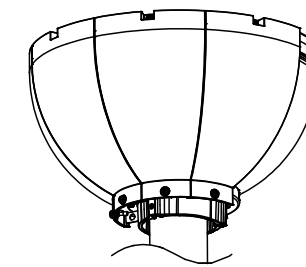
● 器具取付状態 (斜視図) 半球タイプ取付図
