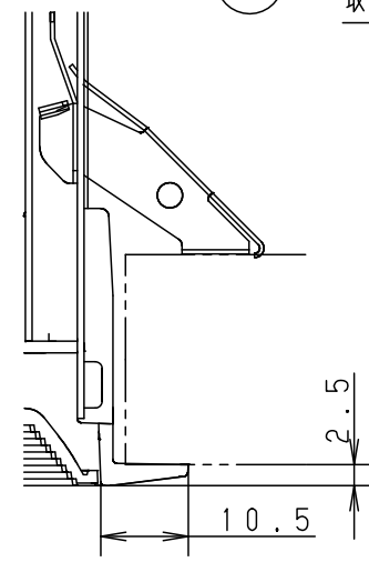
枠部詳細
