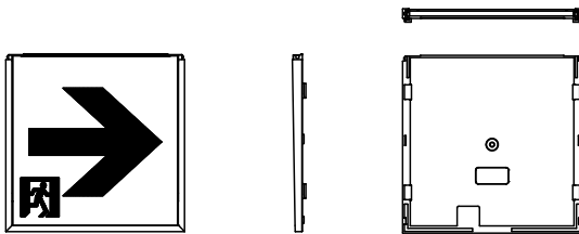
FK20317 (通路誘導灯用表示板)
