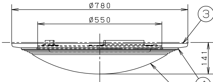
電源ユニット内蔵型
