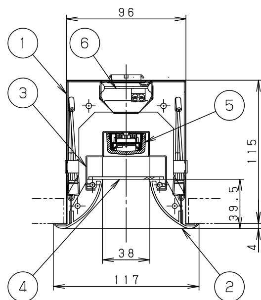
断面詳細図
