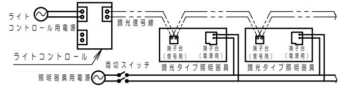
＜結線事例＞ 接地極のない電源に接続する場合
