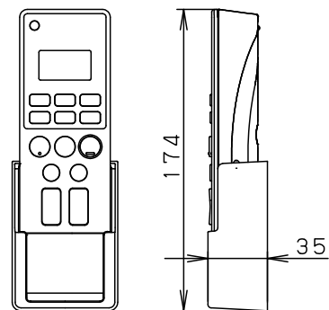
リモコンボックス挿入状態図 (木ネジ2本同梱)
