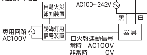
D. 自火報連動による100%点灯あり・消灯なし(2線式配線)の場合
