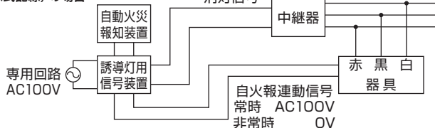
E. 自火報連動による100%点灯あり・信号装置消灯あり(3線式配線)の場合
