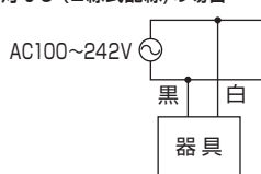
D. 自火報連動による100%点灯あり・消灯なし(2線式配線)の場合
