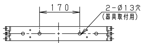
器具取付詳細図
